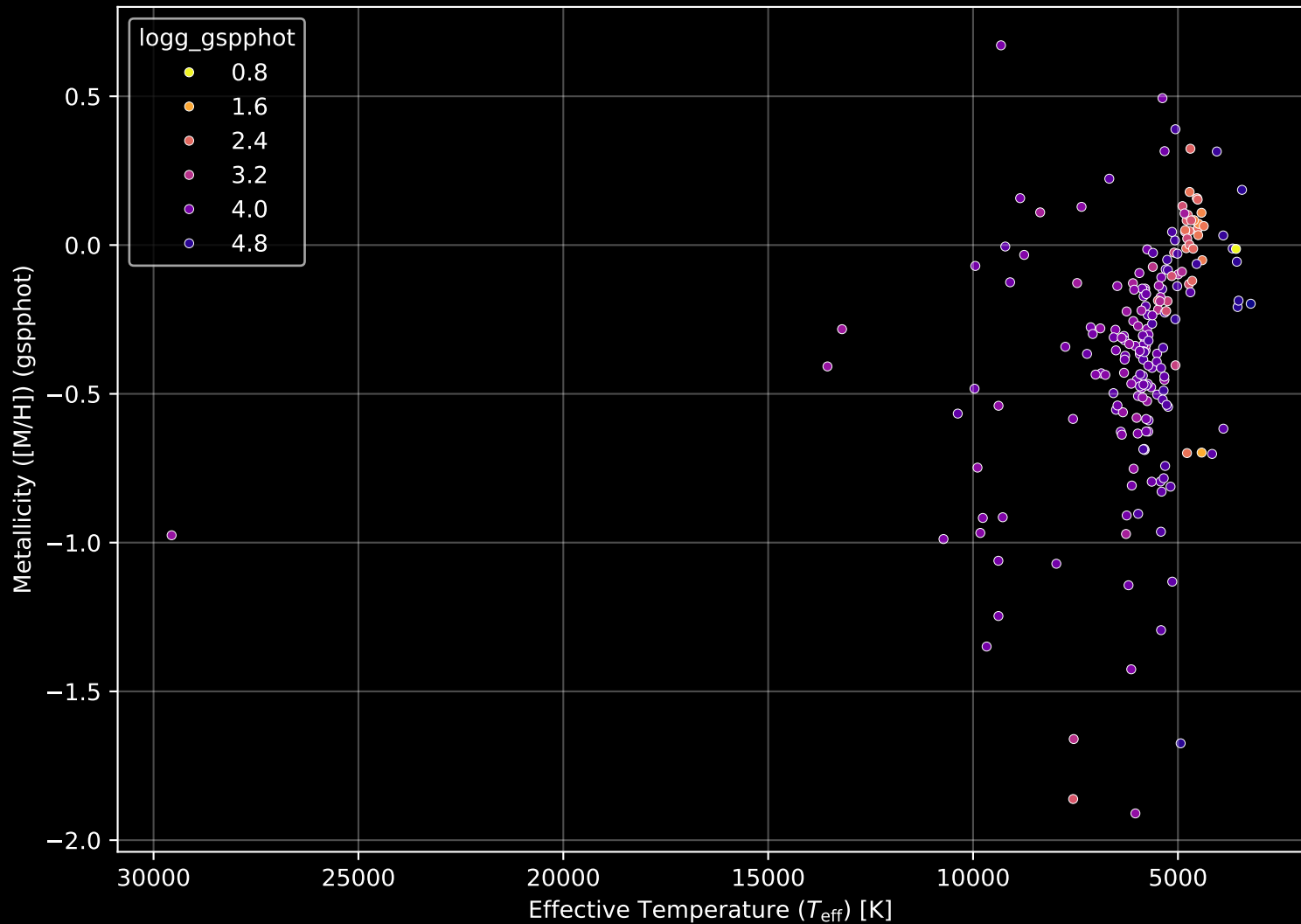
APOGEE DR17 Field: [K2_C7_016-09_btx] Stellar Population Parameters (n= 208)
